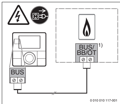
Afb. 8 Aansluiting van de bedieningseenheid op een warmteproducent
