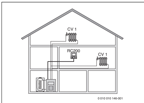
Afb. 1 Voorbeeld voor verwarmingsinstallatie met een cv-circuit CV 1 en RC200 als regelaar (eengezinswoning)
