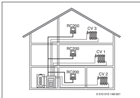
Afb. 3 Voorbeeld voor cv-installatie met drie cv-circuits met telkens een RC200 als regelaar (appartementcomplex)
