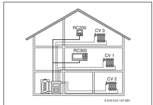
Afb. 2 Voorbeeld voor cv-installatie met drie cv-circuits en RC200 als afstandsbediening (eengezinswoning met aanleunwoning of werkplaats)
