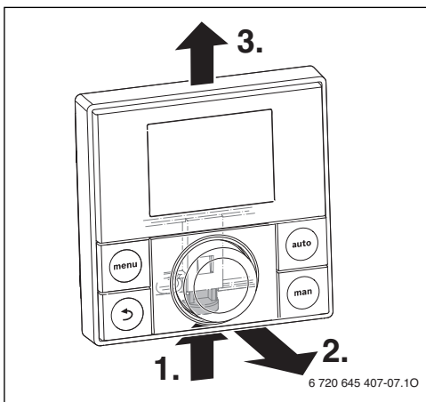
Afb. 10 Bedieningseenheid afnemen
