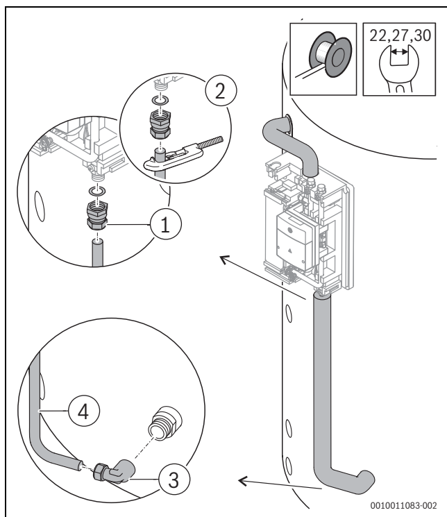
Bild 17 Langes Anschlussrohr des SZ9/7 montieren
