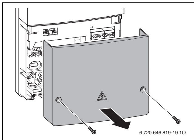
Bild 34 Modul öffnen
