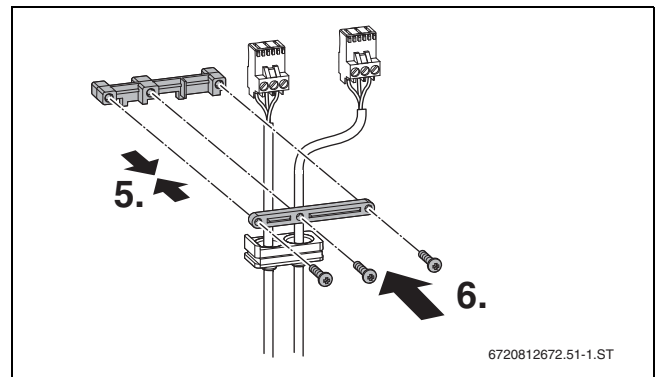
Bild 38 Zugentlastung montieren
