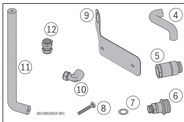
Bild 12 Lieferumfang Speicheranschluss-Set SZ9/7
