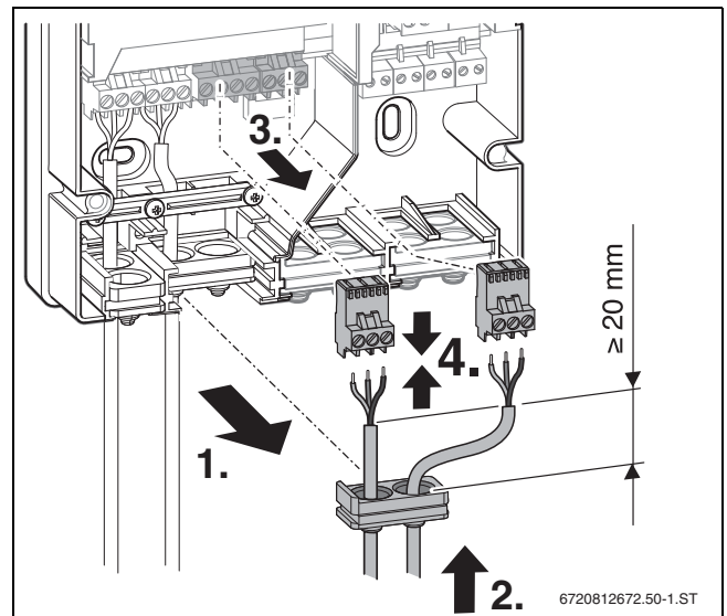
Bild 37 Bauteile an Anschlussklemmen montieren
