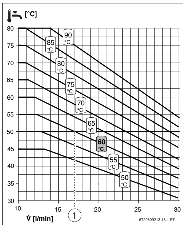
Bild 42 Temperaturverhalten FS/2
