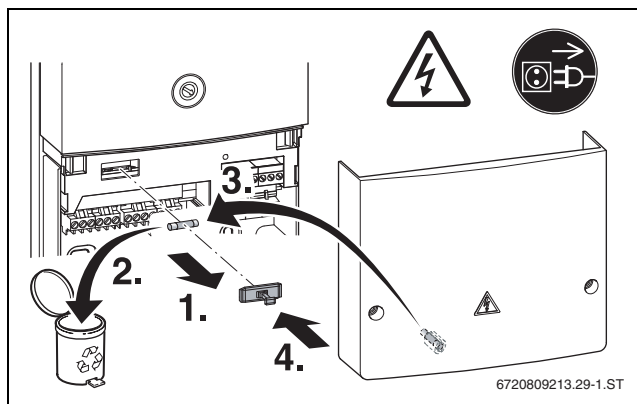
Bild 49 Sicherung tauschen
