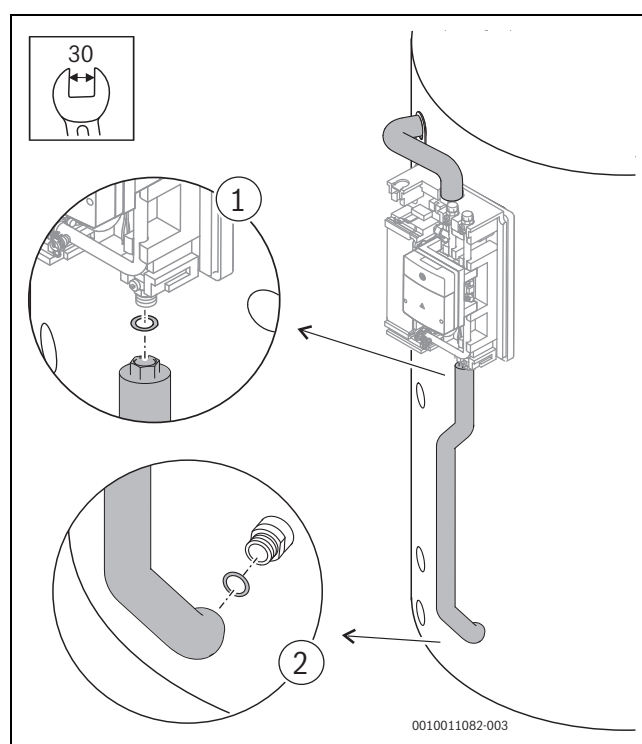
Bild 16 Langes Anschlussrohr des SZ8/7 montieren
