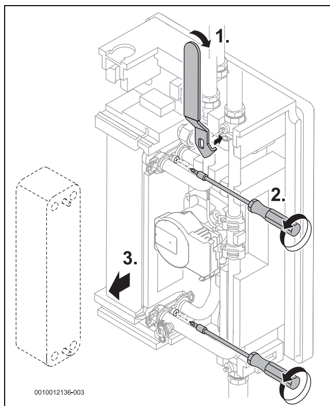
Bild 46 Wärmetauscher demontieren
