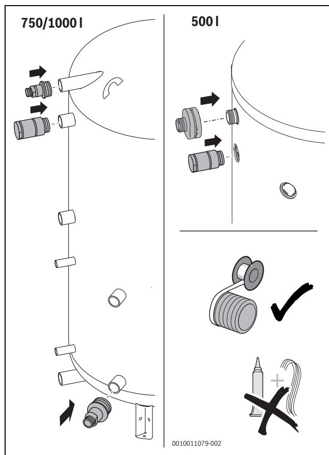
Bild 13 Anschlussstücke einschrauben
