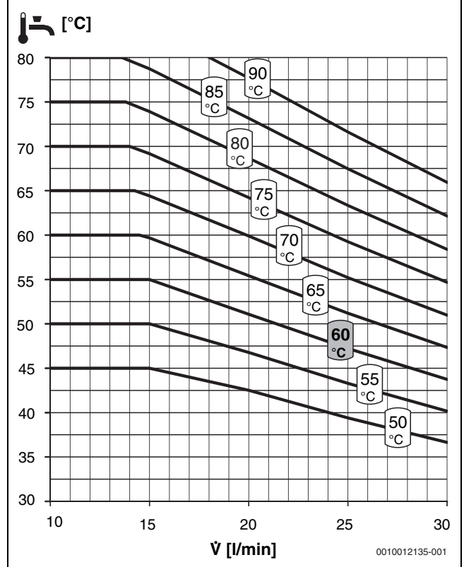
Bild 43 Temperaturverhalten FS20/2
