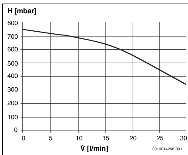
Bild 6 Restförderhöhe Primärkreispumpe
