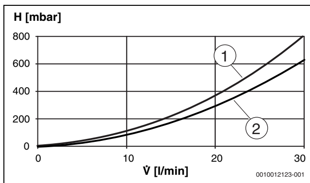
Bild 7 Druckverlust Sekundärseite
