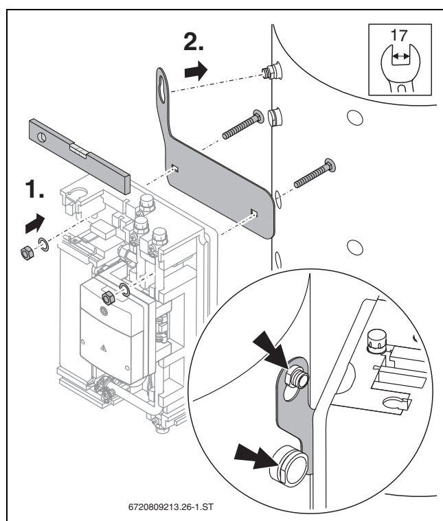
Bild 14 Halteblech (hier: kurz) montieren
