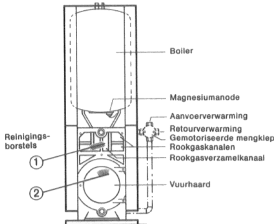
Doorsnede »Loganatherm-Ecomatic« 03.10 TS
