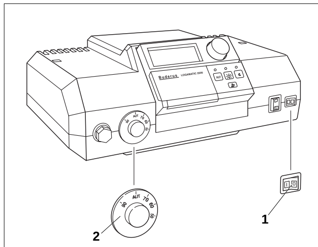
Afb. 1 Regelsysteem Logamatic 2000
